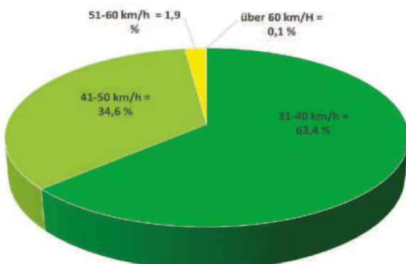
Geschwindigkeiten Kaltbrunner Straße -Höhe Flohzirkus- Richtung Hafnerstraße - 2. Mai bis 2. Juni 2024 Zugelassene Höchstgeschwindigkeit: 50 km/h Fahrzeugzahl gesamt*: 31.422 Fahrzeuge
