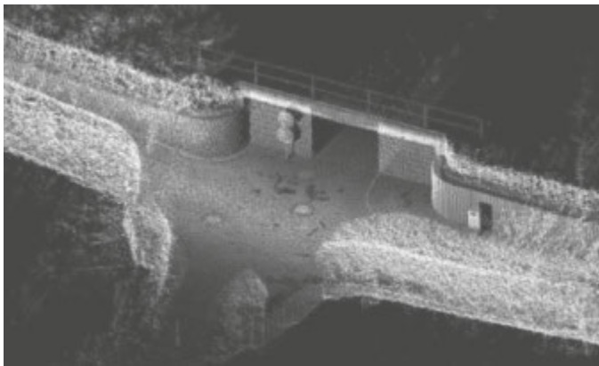
Unterführung Seeweg / Am Kappelhof (sog. „Punktwolke“ aus 3D-Scan)
